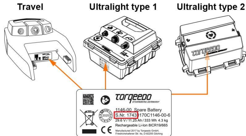
Abb.: Lage des Typenschilds mit Seriennummer
